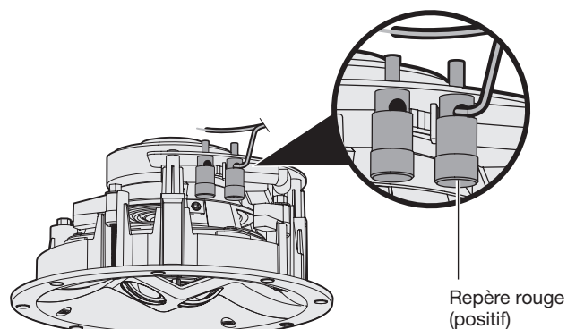
Enceinte Virtually Invisible ® 591
